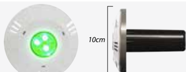
Hiper Led RGB 9W - frontal ABS corpo em ABS, ilumina até 14m 2 , para tubo de 25mm e 50 mm.
